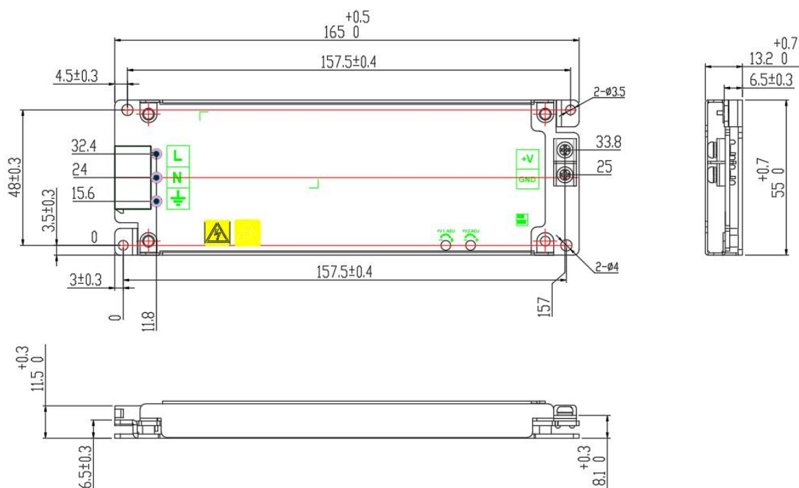
外形尺寸及安装孔——端子坐标图
